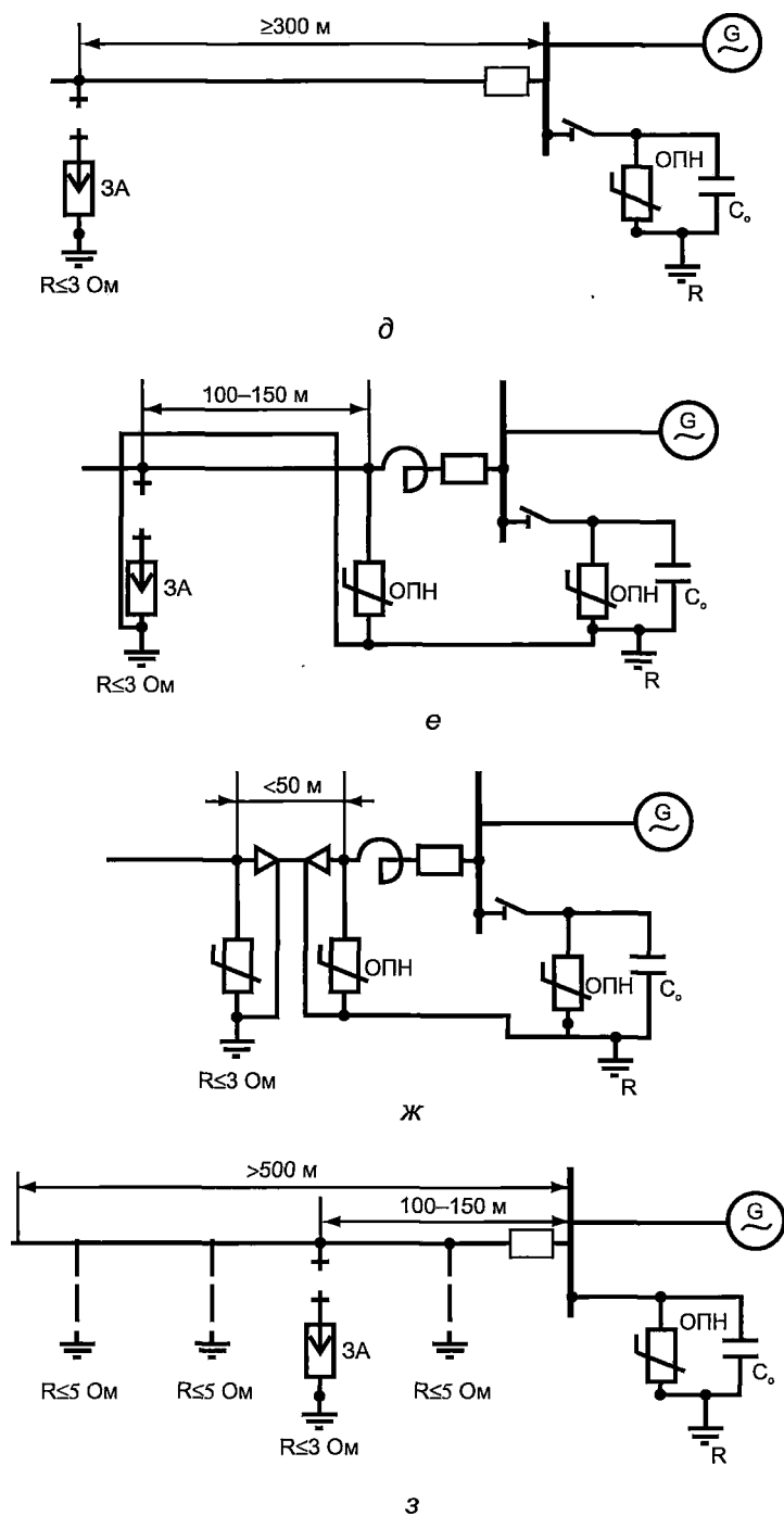
Рисунок 5.2.1, аркуш 2
