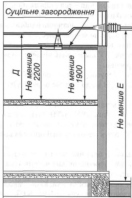
Рисунок 4.2.15 – Найменші відстані від підлоги до необгороджених неізольованих струмовідних частин і нижнього краю фарфору (полімерного матеріалу) ізолятора і висота проходу в ЗРУ. Найменші відстані від поверхні землі до необгороджених лінійних виводів зі ЗРУ поза територією ВРУ та за відсутності проїзду транспорту під виводами
