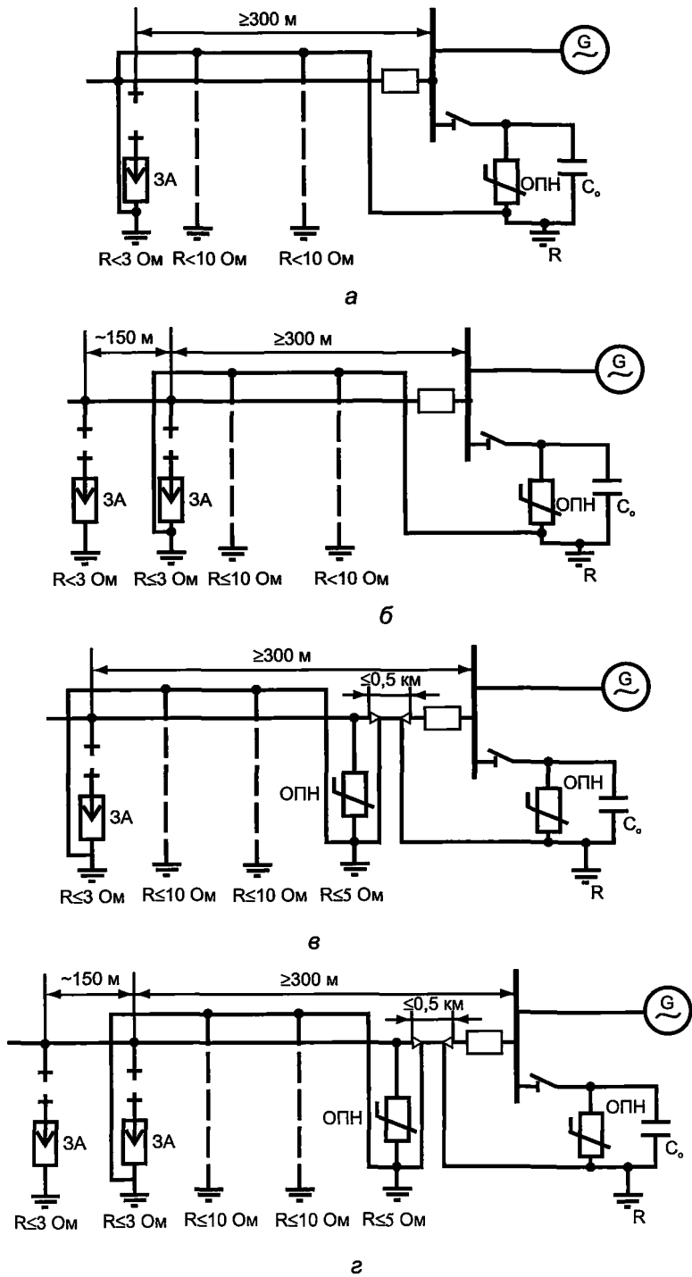
Рисунок 5.2.1, аркуш 1
