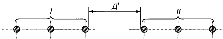
Рисунок 4.2.7 – Найменші відстані по горизонталі між струмовідними частинами різних кіл у разі обслуговування одного кола за невимкненого іншого
