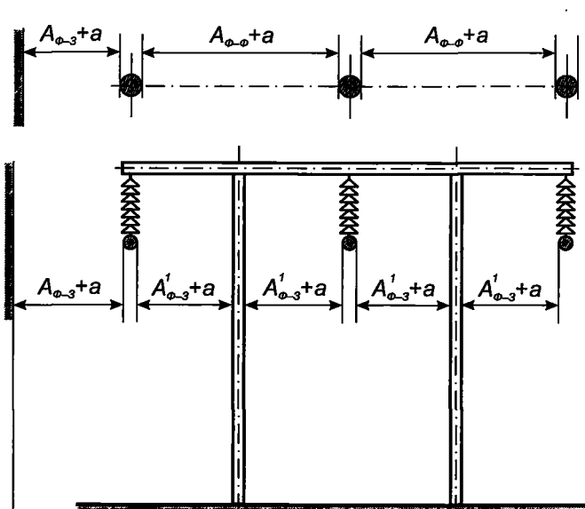
Рисунок 4.2.2 – Найменші відстані в проєкті за гнучких неізолюваних шин між струмовідними і заземленими частинами та між струмовідними частинами різних фаз, розташованими в одній горизонтальній площині
