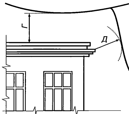
Рисунок 4.2.10 – Найменші відстані між струмовідними частинами та будівлями і спорудами
