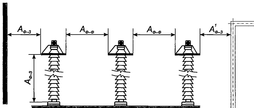
Рисунок 4.2.1 – Найменші відстані в проєкті за жорстких шин між струмовідними і заземленими частинами ( A_{Ф-З} , A'_{Ф-З} ) та між струмовідними частинами різних фаз ( A_{Ф-Ф} )
