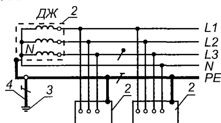
нейтраль розподілено
