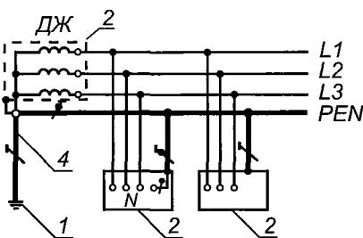
Система TN-C
