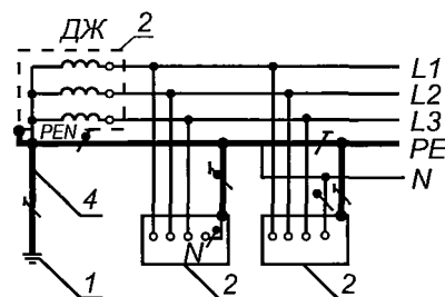
Система TN-C-S
